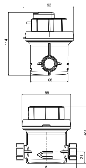
Wymiary
