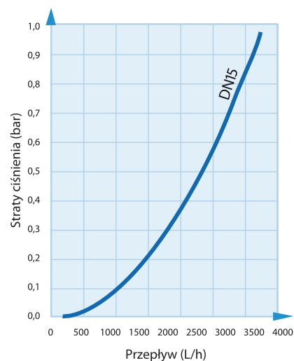
Straty ciśnienia wodomierza Aquadis+ PE
